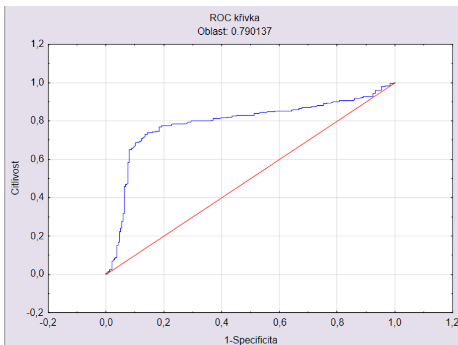
Obrázek 1 ROC křivka
