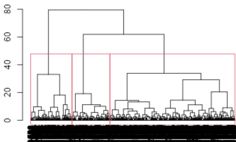
Obrázek 1: Dendrogram hierarchické shlukové analýzy.
