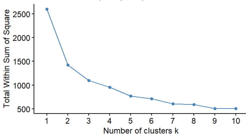
Elbow metóda pre výber počtu klastrov
