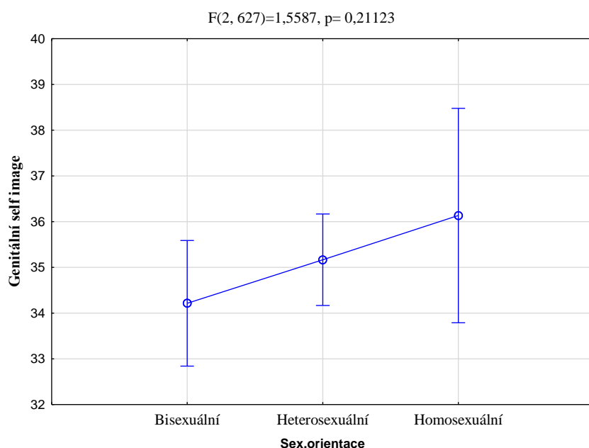
Graf 1: Vztah mezi genitálním self image a sexuální orientací
